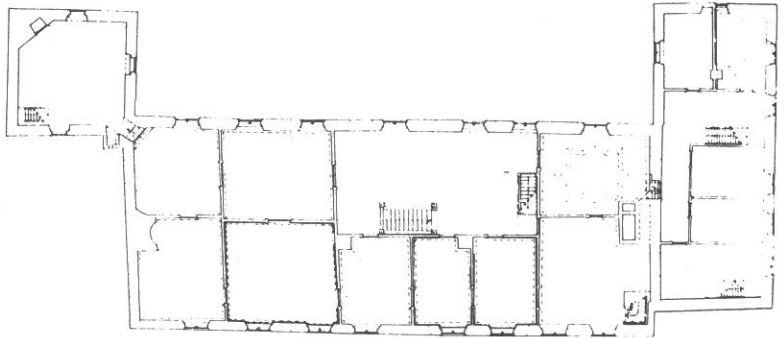
Fig. 20 Opmåling af 2. etagen. Mål 1:200
